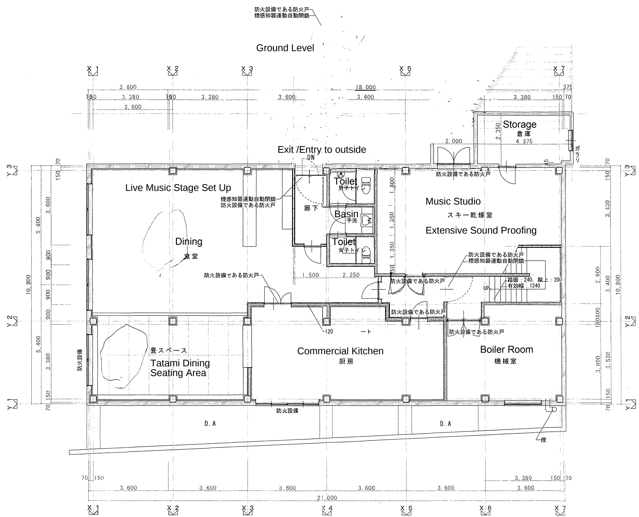
地下1階平面図 S = 1 : 100 Basement Level
