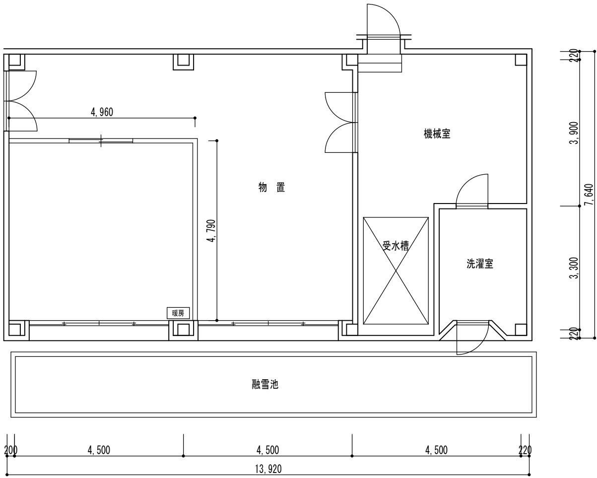
改修平面図 S : 1 / 100
